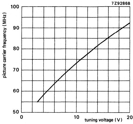
Fig. 10 Low v.h.f. band.
