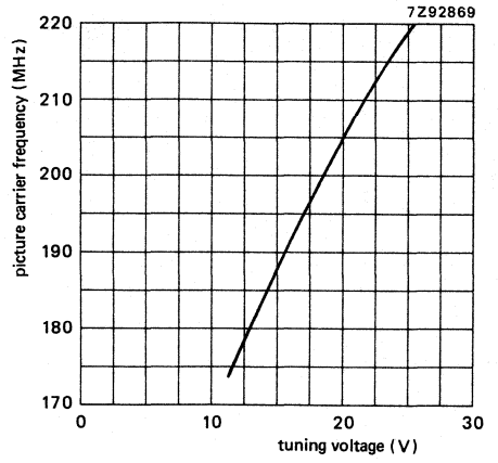
Fig. 11 High v.h.f. band.
